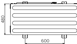
HORNÍ POHLED
