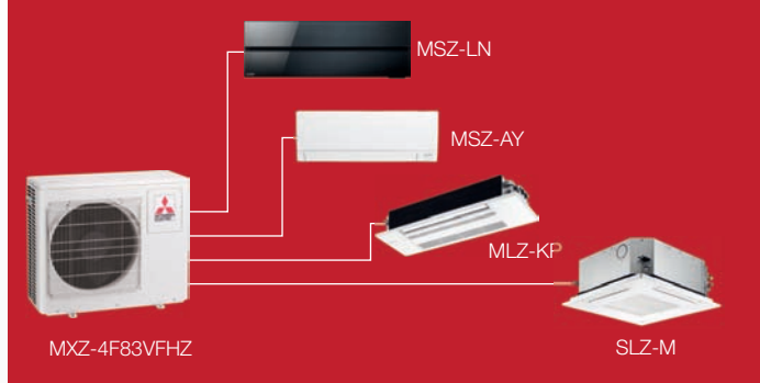
Príklad napojenia jednotky MXZ-4F83VFHZ
