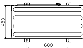
HORNÍ POHLED
