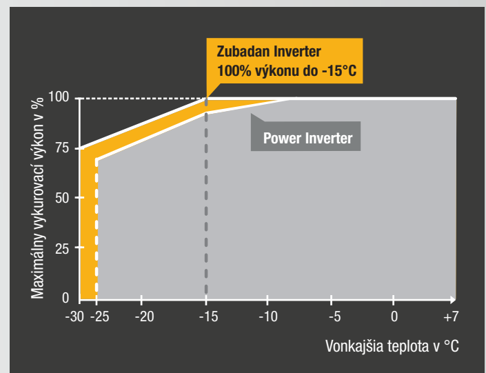
Graf závislosti výkonu od vonkajšej teploty
