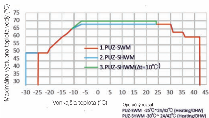
Graf závislosti výstupnej teploty vody od vonkajšej teploty
