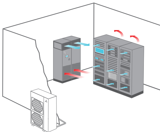
Klimatizační skříně s-MEXT v provedení „Over“ s volitelným ventilačním otvorem pro výstup vzduchu
